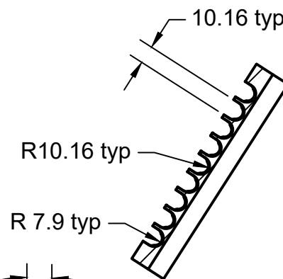
SECTION A-A SCALE 1:3
